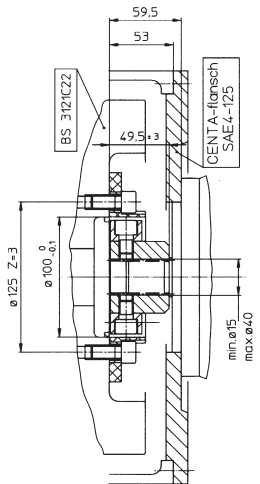
CF-K-100-100 Perkins Serie 500
